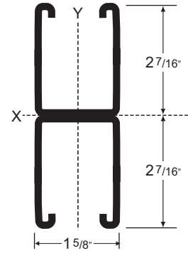
D-12A
