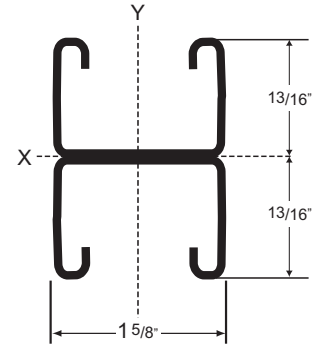
C-14A
