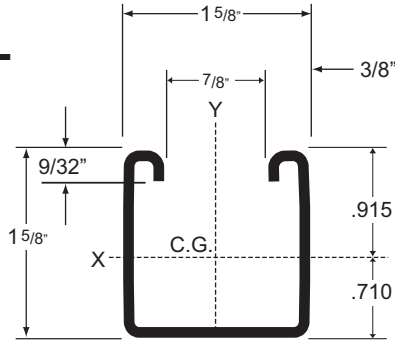
A-14
