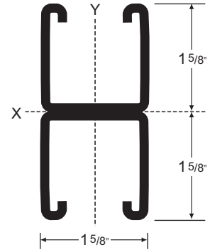
A-12A
